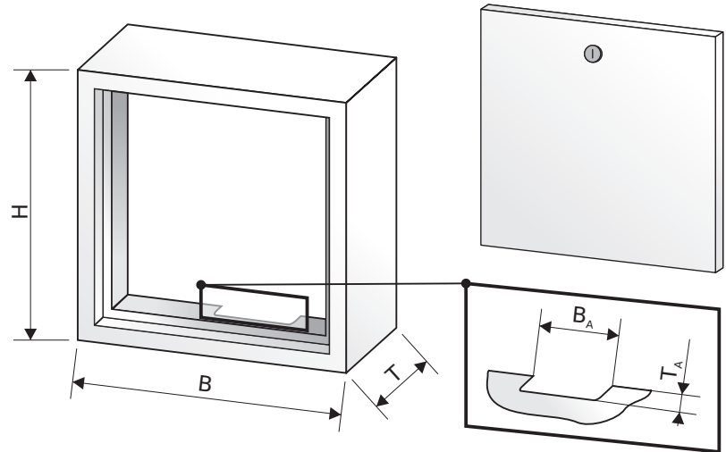
Ausschnitt A für Kabeleinführung
