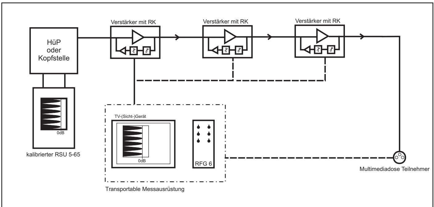
Schema: Rückkanal einstellen und prüfen in BK-Anlagen mit RSU 5-65 und RFG 6
